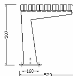
vista lateral 1/10
