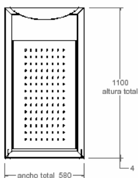
vista alzado 1:20
