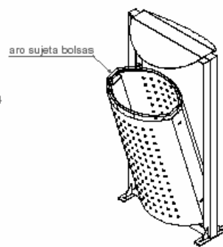
detalle papelera abierta 1:20
