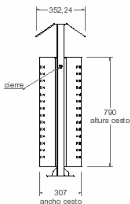
vista lateral 1:20
