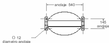
vista en planta 1:20
